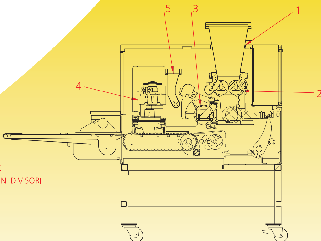
SEZIONE A-A
